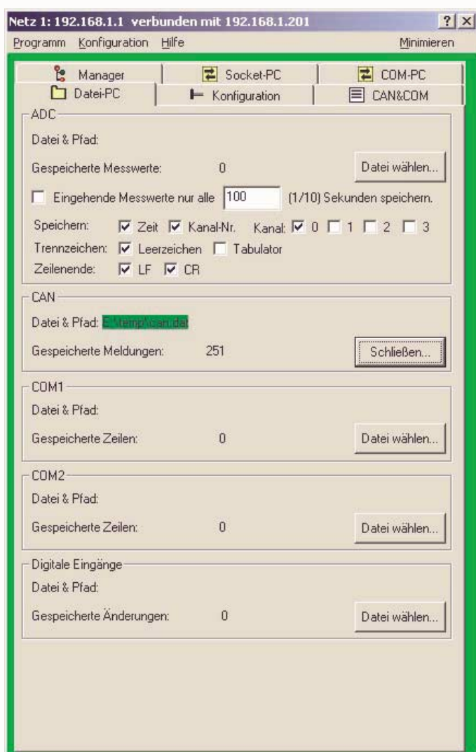
Abb. 18: Dialogbox Datei-PC
