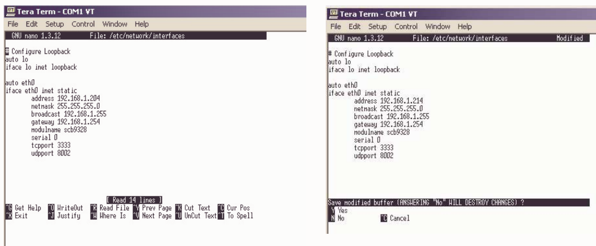
Abb. 25: Der Editor „nano“ beim Editieren (links) und beim Speichern der Datei (rechts)
