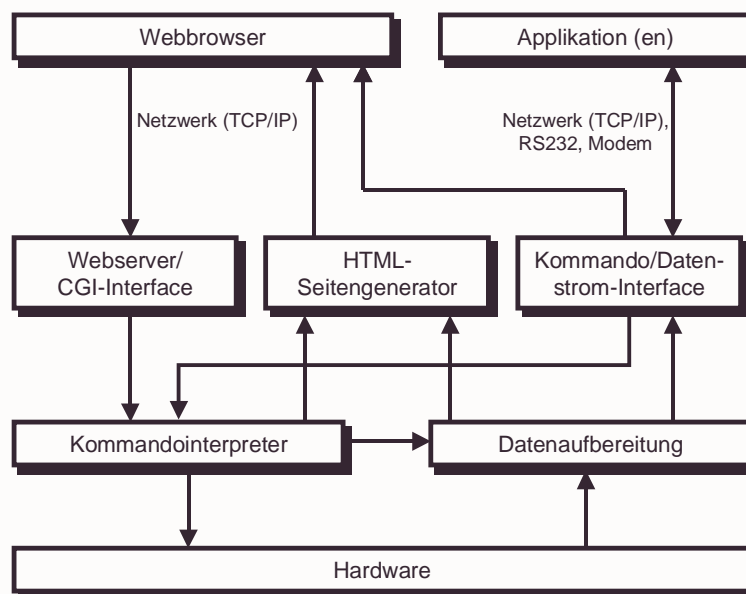
Abb. 21: Kommunikationszugriff (vereinfacht)
