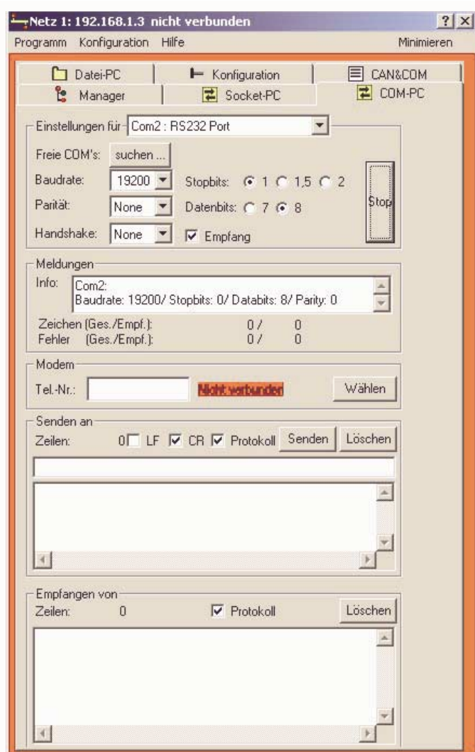
Abb. 16: Dialogbox COM-PC
