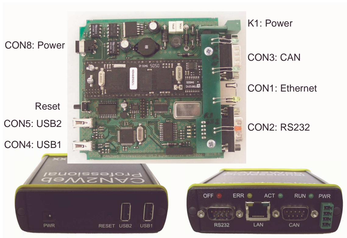
Abb. 30: Steckverbinder CAN2Web-Professional
