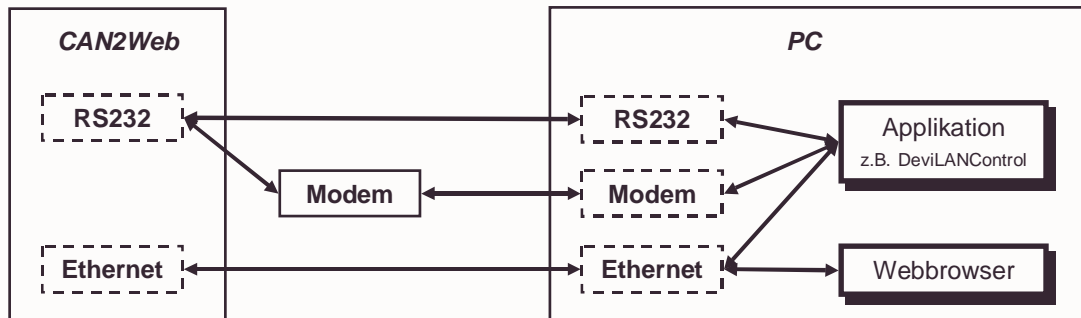
Abb. 20: CAN2Web Kommunikationsschnittstellen
