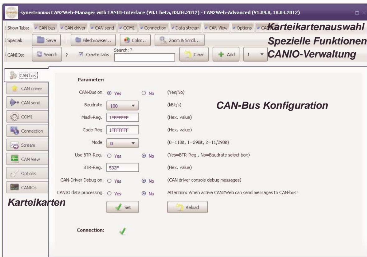
Abb. 8: CAN2Web qooxdoo-Interface, Menüführung und Bedienung über Webbrowser
