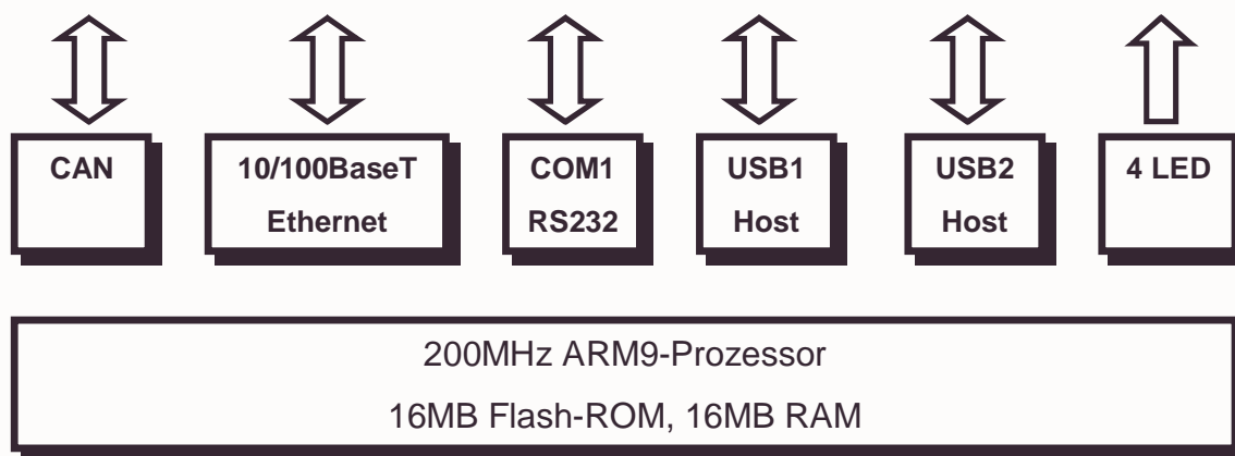
Abb. 4: Hardwareübersicht CAN2Web-Professional
