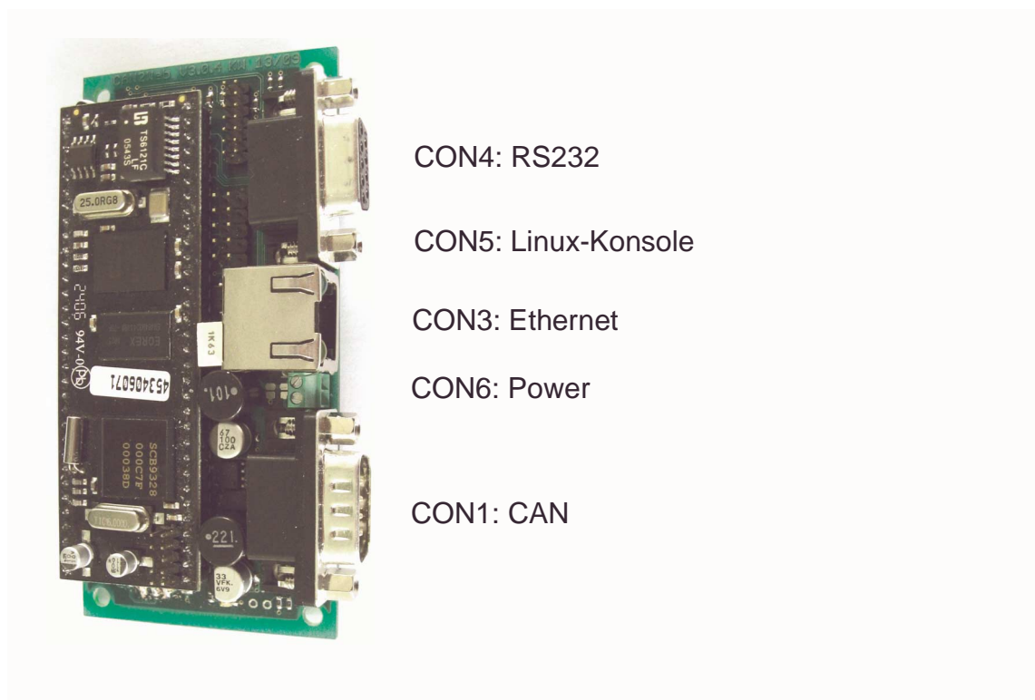
Abb. 29: Steckverbinder CAN2Web-Advanced
