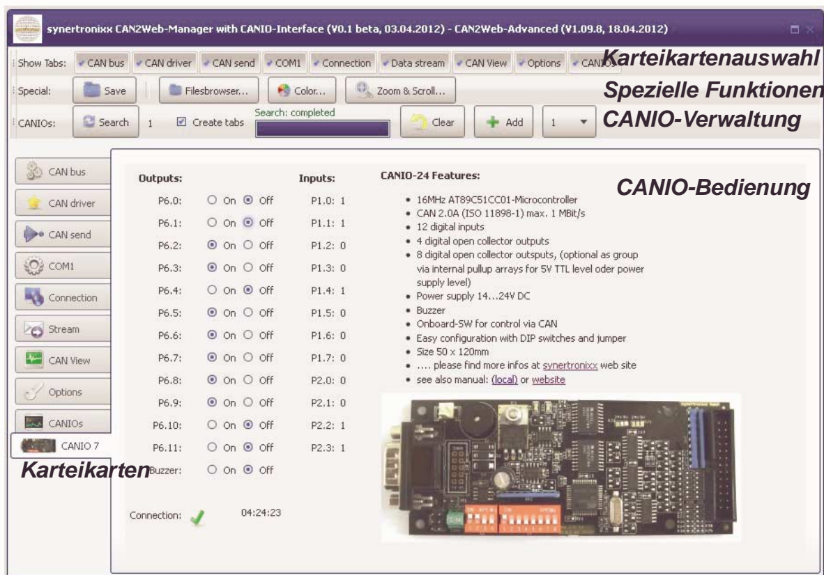
Abb. 10: CAN2Web qooxdoo-Interface, Bedienung von CANIO-Modulen
