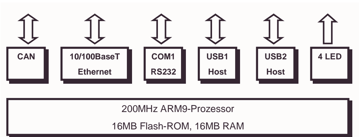
Abb. 3: Hardwareübersicht CAN2Web-Advanced
